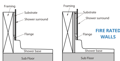
FLANGE DETAILS (U.S.)
