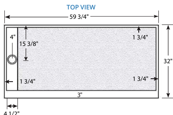
FLANGE DETAILS (U.S.)
